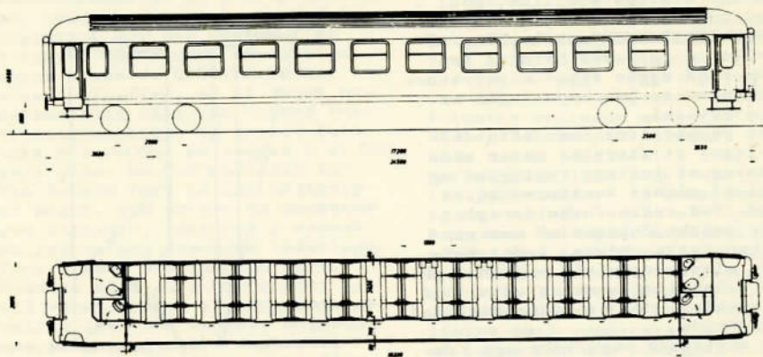
Skitse af den nye 2. kl. standardpersonvogn. Vognen bliver 24,5 m lang over pufferne, vil rumme 10 ku- kupeer med i alt 80 pladser og få særskilte rum for håndvaske
