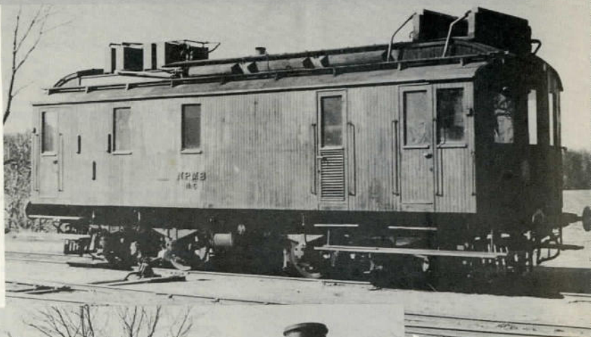
NPMB's motorvogn M 6. Foto: KWH.
