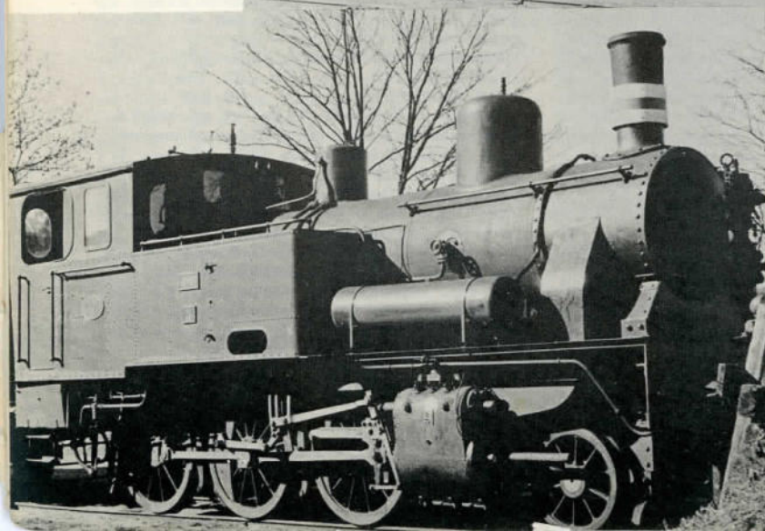
Omflakkeren NPMB 3. foto: KWH.
