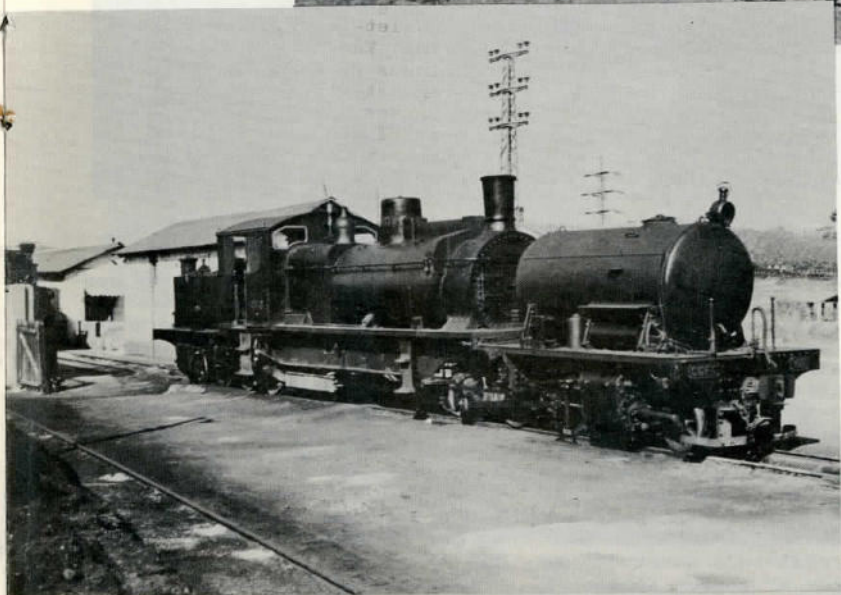
Fig.4. CFGL Mowres (Alta) St. Leonard, Belgien. Foto:OWL.
