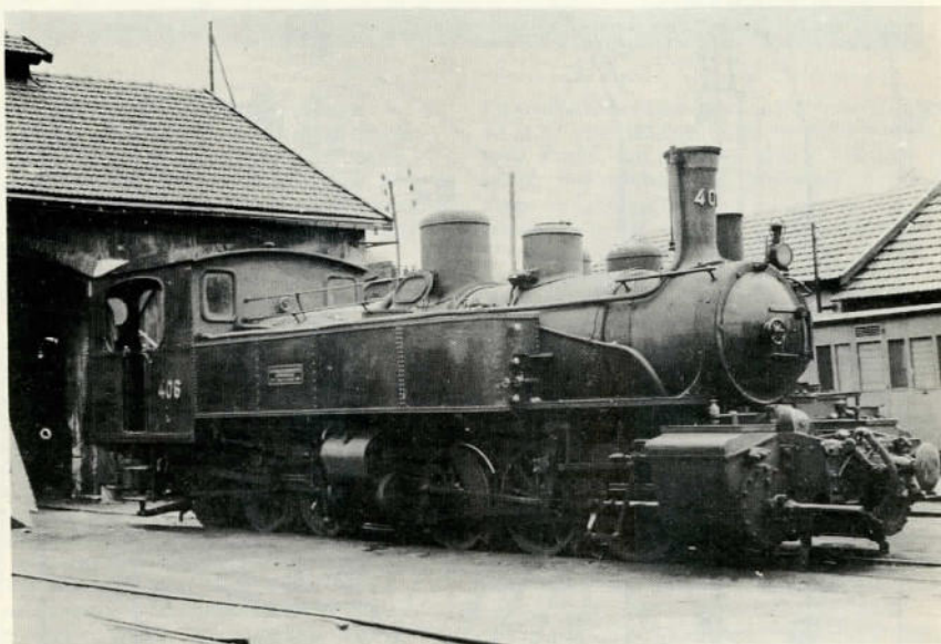
Fig.1. CFD Réseau du Vivarais le Cheylard 1958, 1000 mm sporvidde. Foto: O.W.Laursen.
