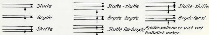
Fig. 18. Eksempler på kontaktkombinationer til telefonrelæer.
