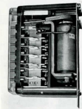
Fig. 25. Op-skåret RC-relæ.
