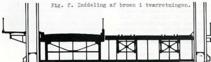
Fig. f. Inddeling af broen i tværretningen.
