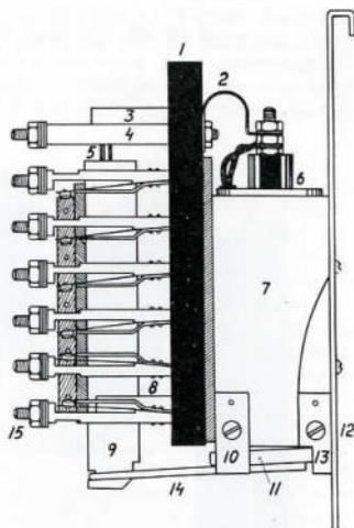
Fig. 20. Centralapparatrelæ type RA. 1: Bundplade f. kontaktsystem 3: Tapleje 4: Spoletilslutningssklemme 5: Styretap 6: Magnetpol 7: Magnethus 9: Lineal 10: Ankerstop 11: Anker 15: Kontaktstøtte.
