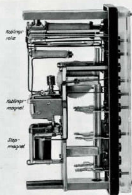
Fig. 24. Tidsrelæ.
