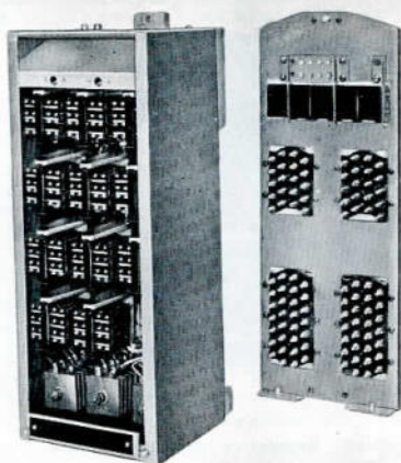
Fig. 29. Relægruppe.
