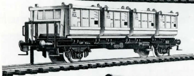
Containervogn af typen Eoskrt
