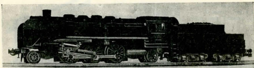
PIKO's nye HO-lok, model af Reihe 23 (DR), samt herunder motoraggregatet
