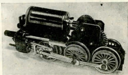
PIKO's nye HO-lok, model af Reihe 23 (DR), samt herunder motoraggregatet
