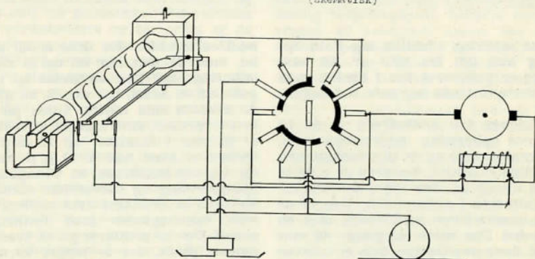
Skitse over polariseret relæ og den elektriske forbindelse.
