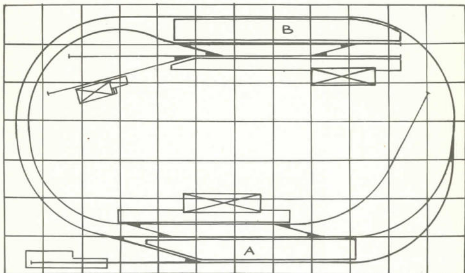
Fig. nr. 1 viser en videreudvikling af den for begynderen så kendte skinneoval. Station A er både overhalingstation og forgretningsstation for sidebanen — med endestation på sydsiden af station B. Til skala HO svarer hvert kvadrat til 20x20 cm.
