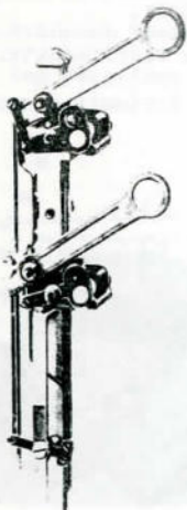
Fig. 1 - detaille af nyt signal 446/13.
